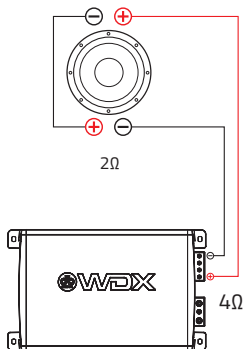
1 X 2Ω DVC SUBWOOFER 2Ω
