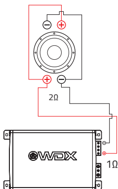
1 X 2Ω DVC SUBWOOFER 2Ω
